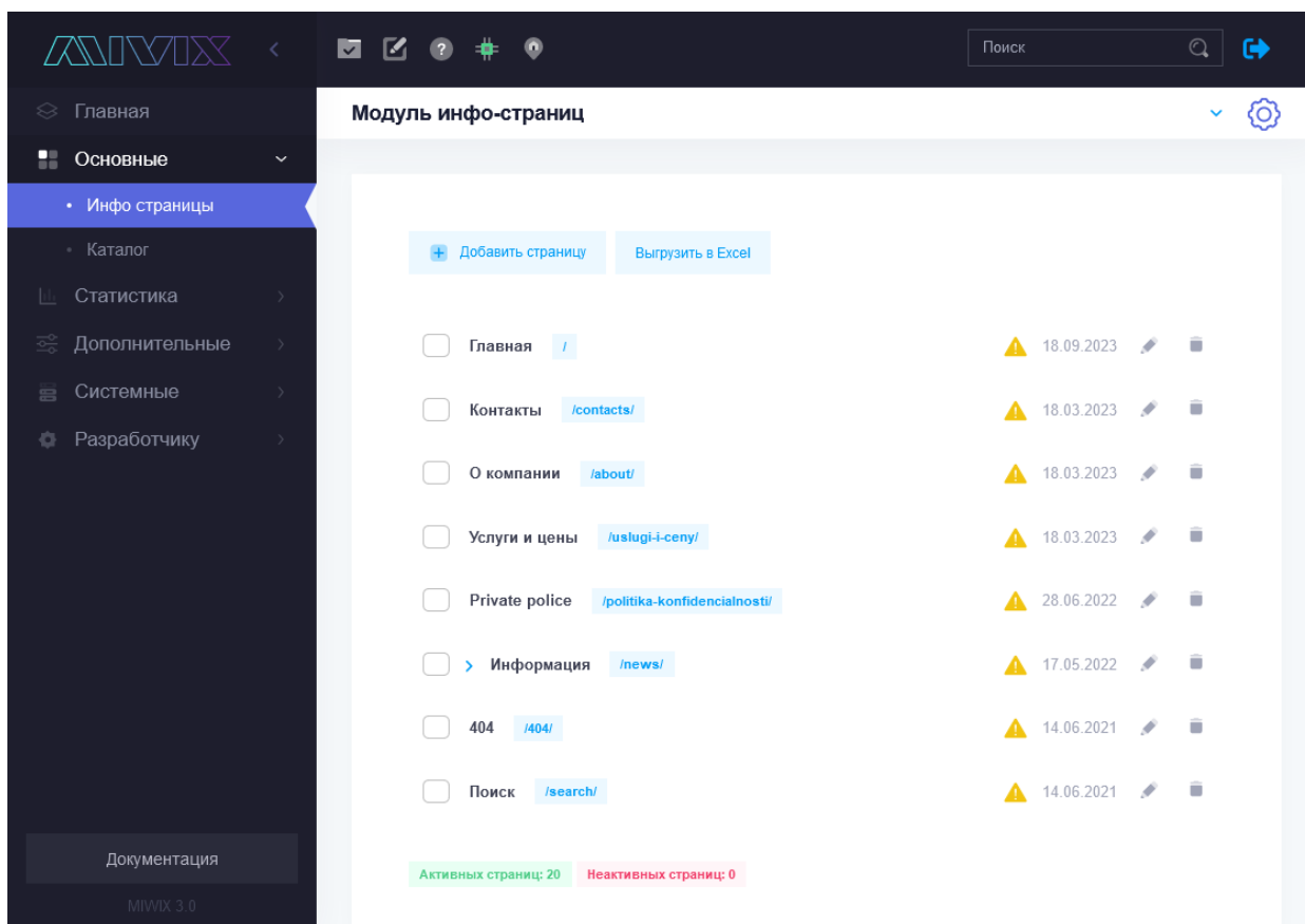
Рис. 4. Модуль инфо-страниц
