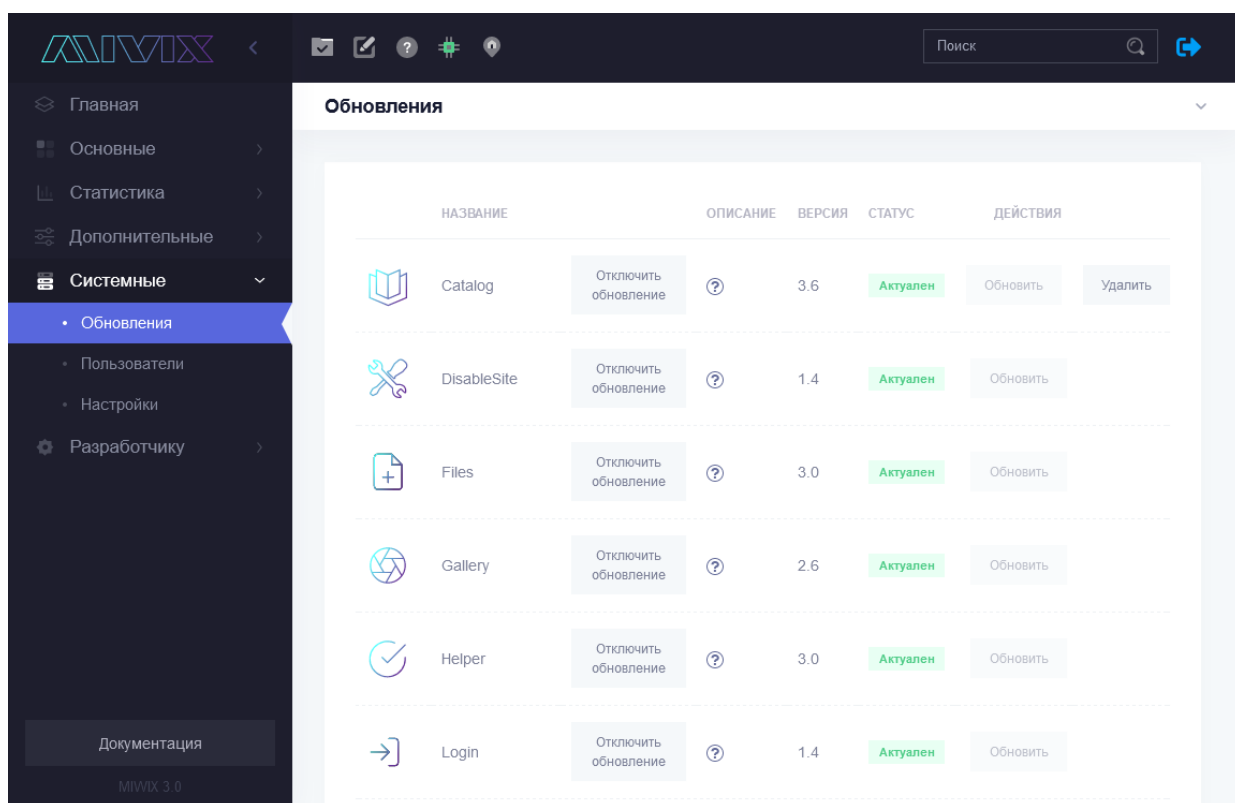
Рис. 5. Обновления MIWIX.
