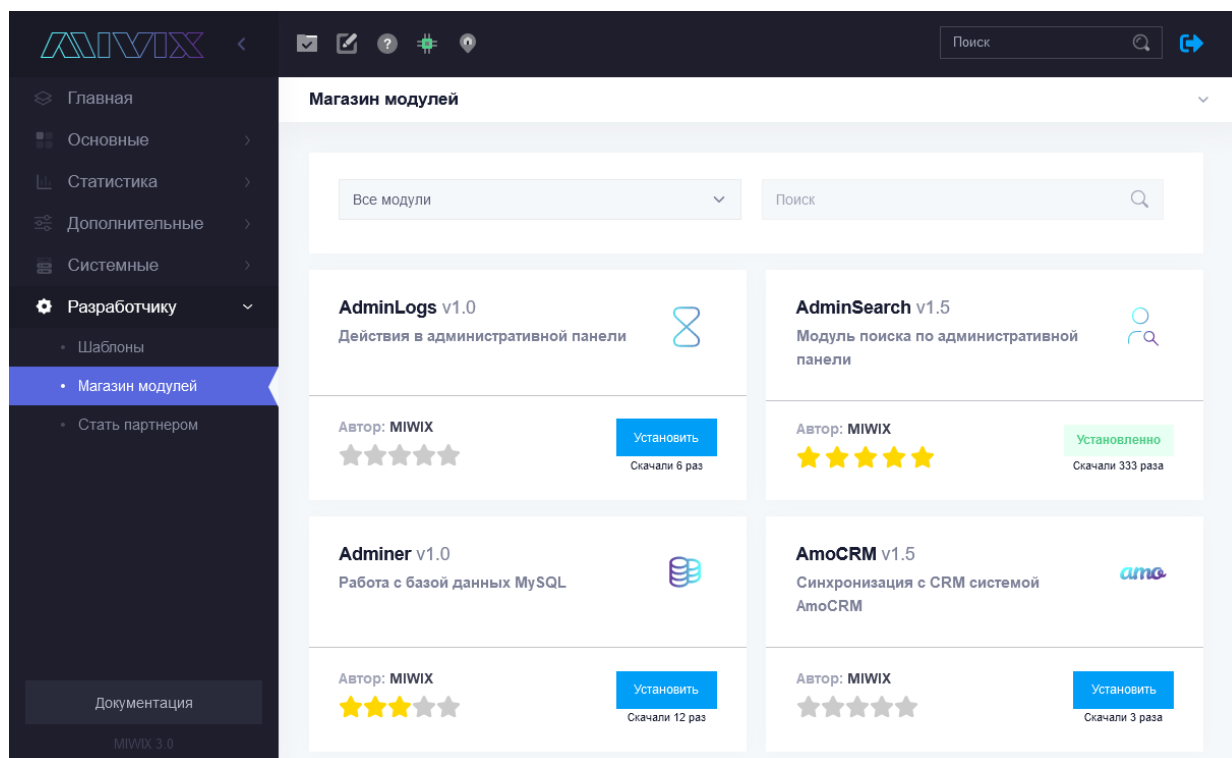
Рис. 7. Магазин модулей.
