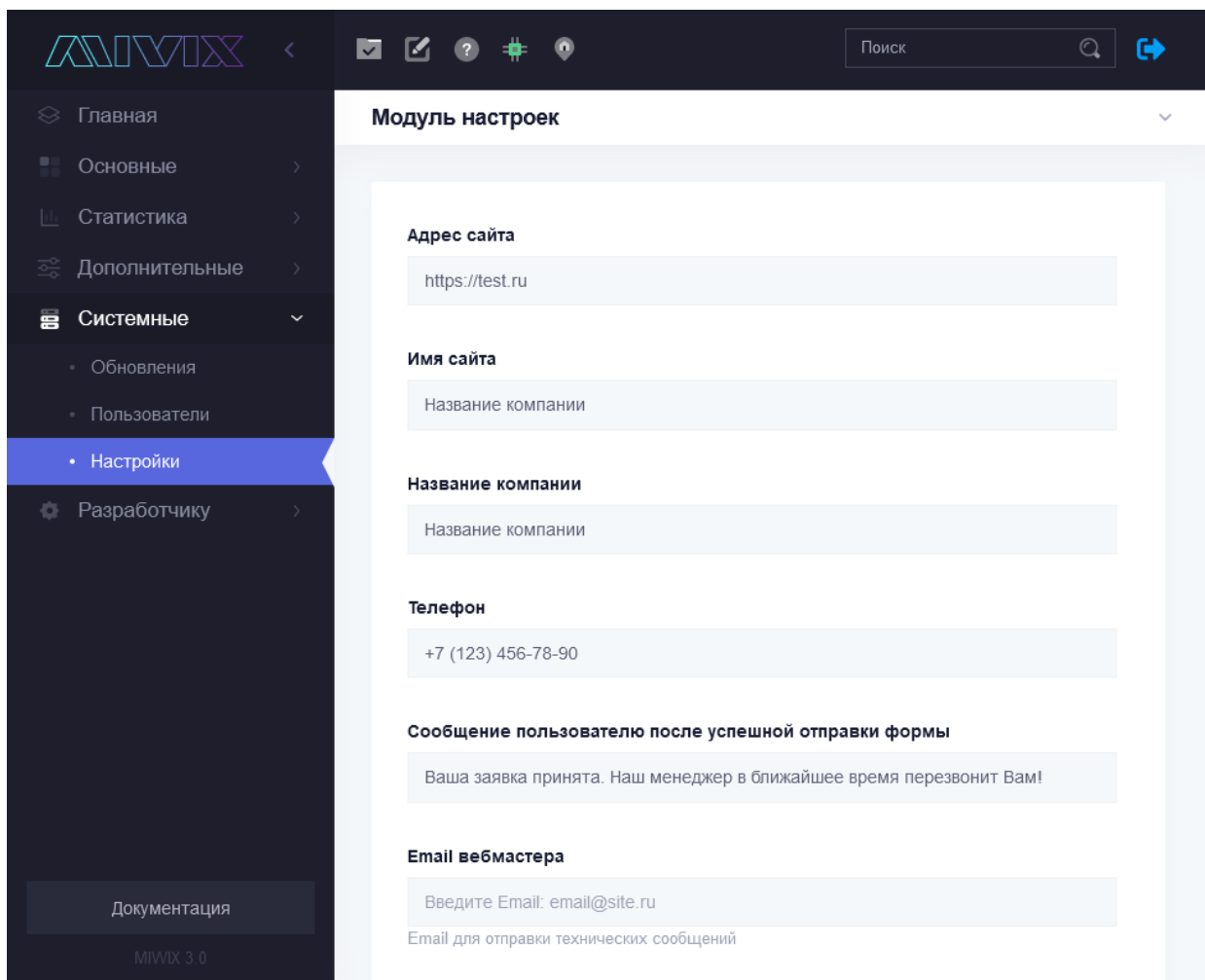
Рис. 3. Системные настройки
